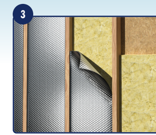
3 Exterior Wall* / Mur extérieur* / Pared exterior*
