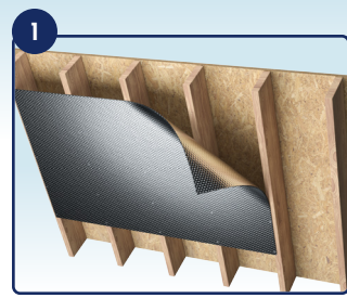
1 Attic / Grenier / Ático
