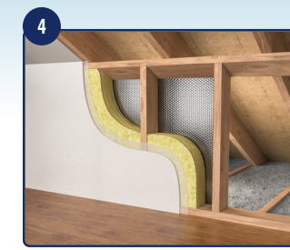
4 Knee Wall* / Mur bas* / Estructura de soporte para vigas*
