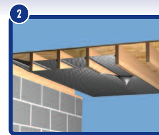
Crawl Space / Vide sanitaire / Entresuelo
