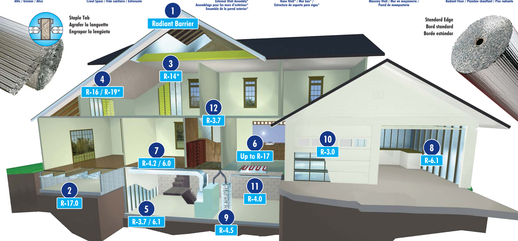
Attic / Grenier / Ático
