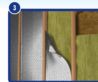
External Wall Assembly* Assemblage pour les murs d'extérieur* Ensamble de la pared exterior*
