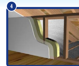
Knee Wall* / Mur bas* / Estructura de soporte para vigas*
